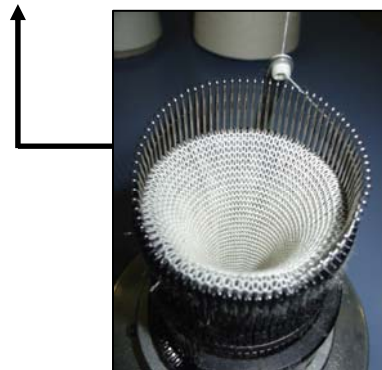
Maille fabriquée sur circulaire de trame
